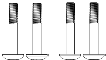
Vite×4 (M8*60*20)
